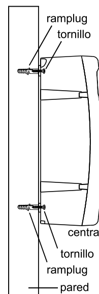
figura 6: fijación en la pared
