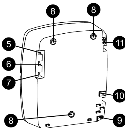
figura 2: gabinete - vista trasera
