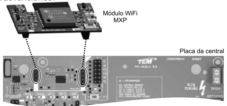
Figura 12: Instalación del módulo MXP
