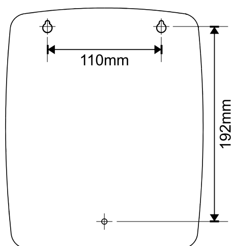
figura 4: Plantillade fijación
