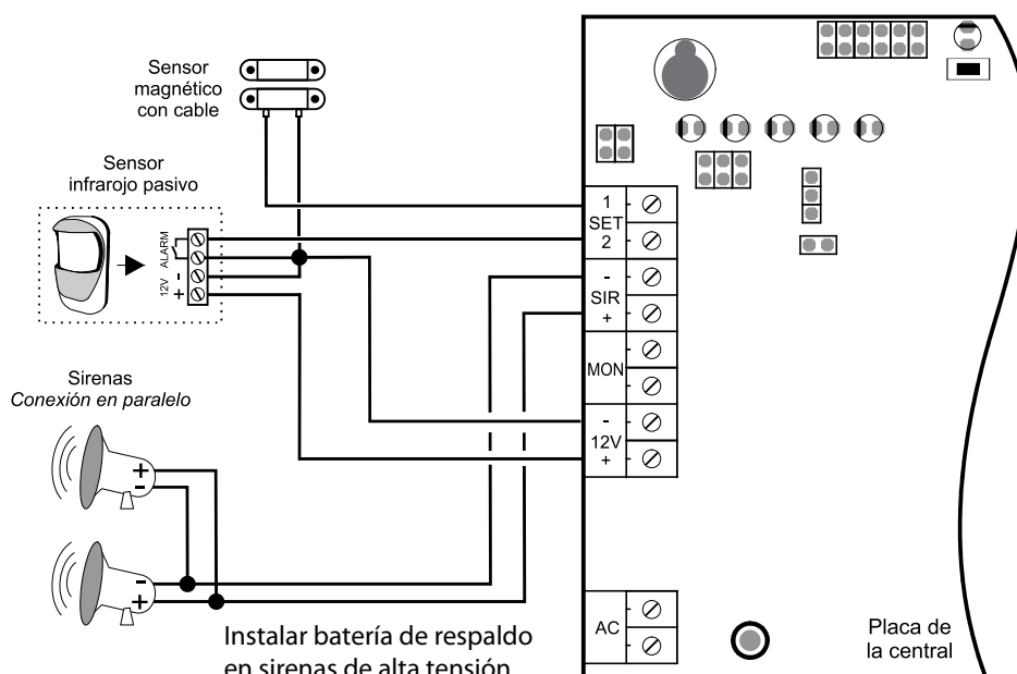
Figura 11: Conexión de sirenas y sensores
