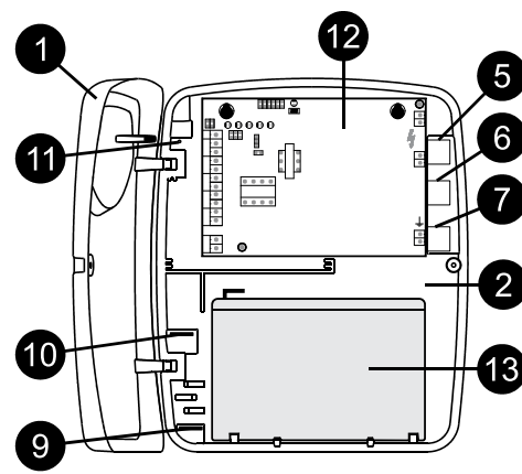
figura 3: partes internas
